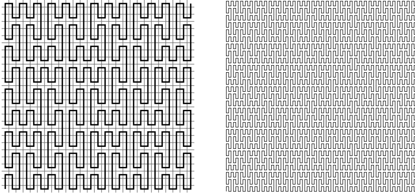
Figur 4: Tredje og fjerde tilnærming til Peano-kurven.
