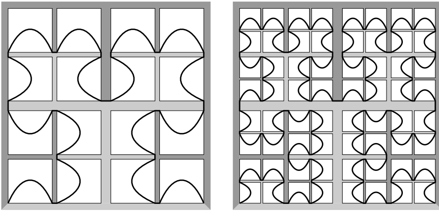
Figur 7: Annen og tredje tilnærming til Hilbert–Osgood-kurven.
