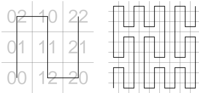
Figur 3: Første og annen tilnærming til Peano-kurven.
