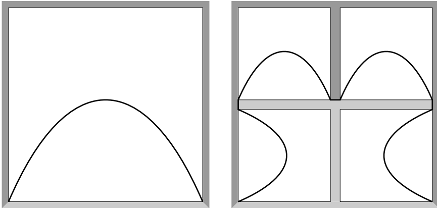
Figur 6: Nullte og første tilnærming til Hilbert–Osgood-kurven.
