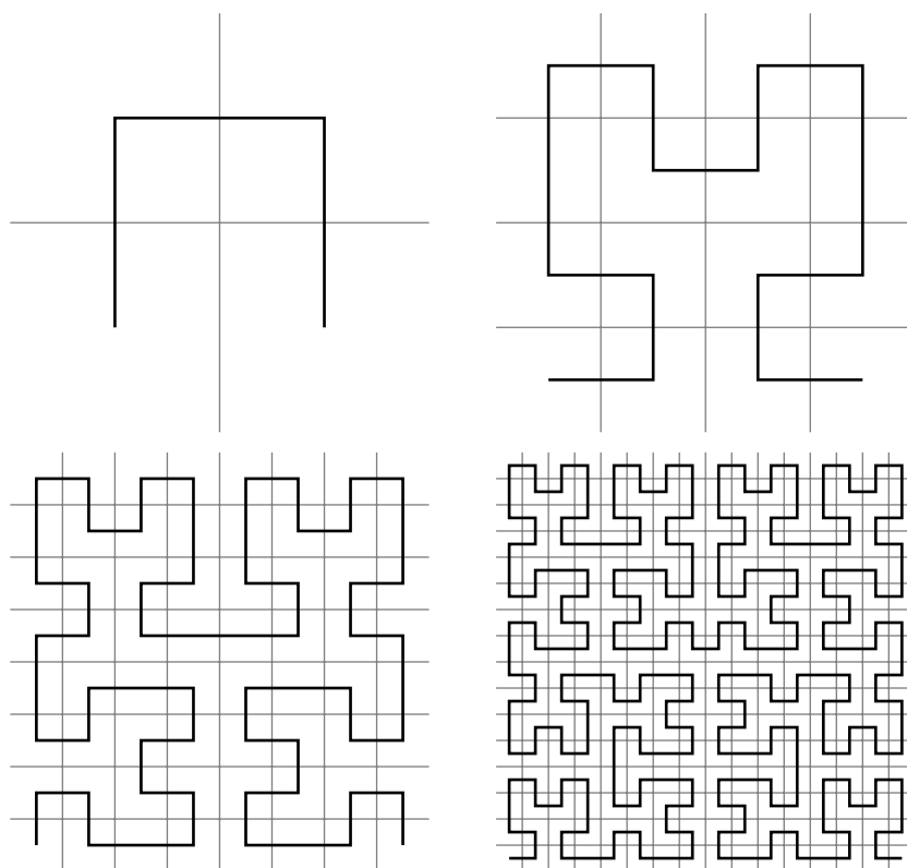
Figur 5: Første til fjerde tilnærming til Hilbert-kurven.
