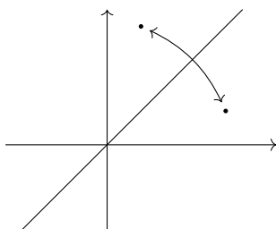
Matrisen A reflekterer vektorene om diagonalen (vektorer markert som \cdot )
