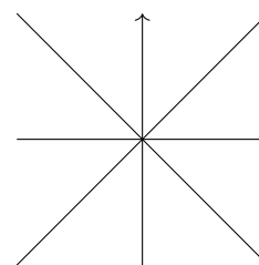
Ortogonale egenrom for A
