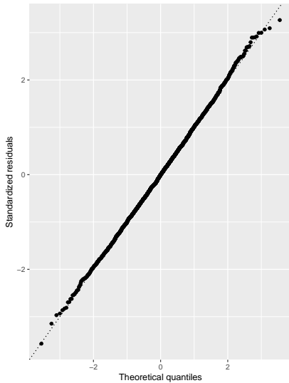
Normal Q-Q
