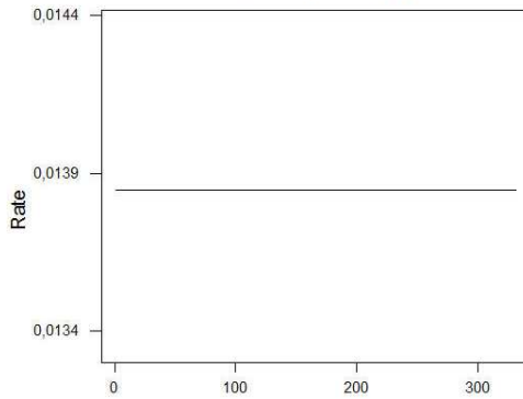
Hazard Function
